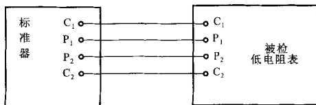
图1 整体检定原理图
